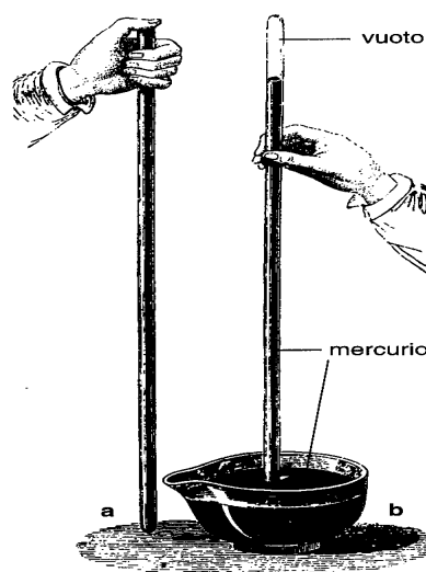
Figura 2: Barômetro de Torricelli. Fonte: (OLIVEIRA, 2009, p.19)
